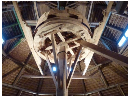
Pferdegöpel in Johanngeorgenstadt
